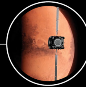
2. MARS SWINGBY
