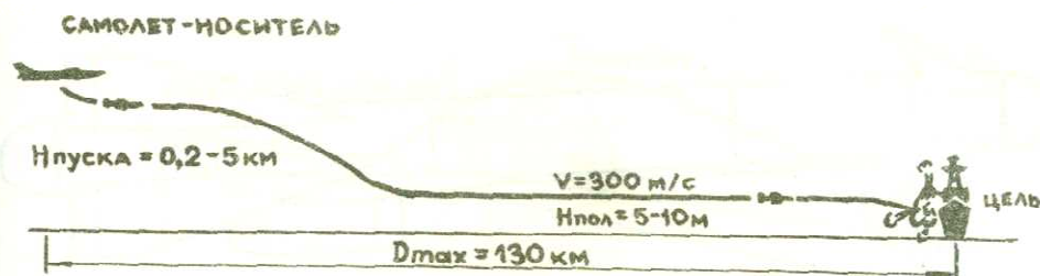
Схема боевого применения ПКР Х-35 (АС-17).
