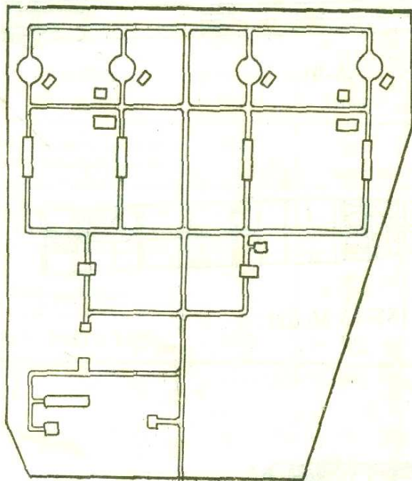
Схема размещения ракетного полка с наземными пусковыми установками ракет Р-12У.
