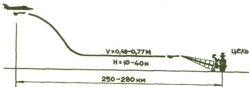
Схема боевого применения ПКР X-65C.
