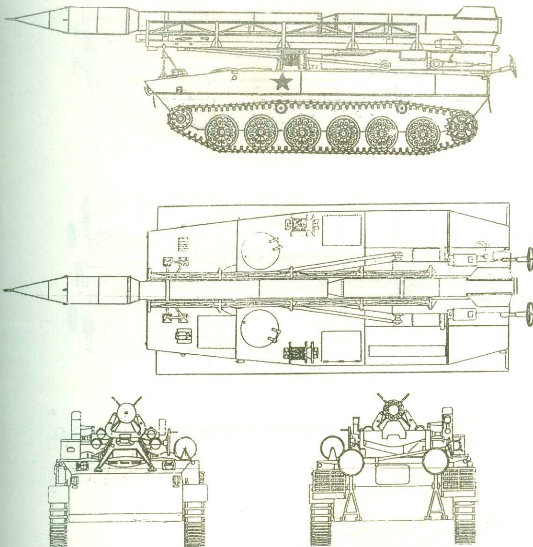
Пусковая установка и ракета комплекса "Луна" (FROG-3).
