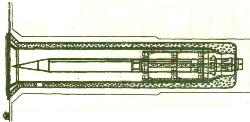
ШПУ ракеты Р-12У.
