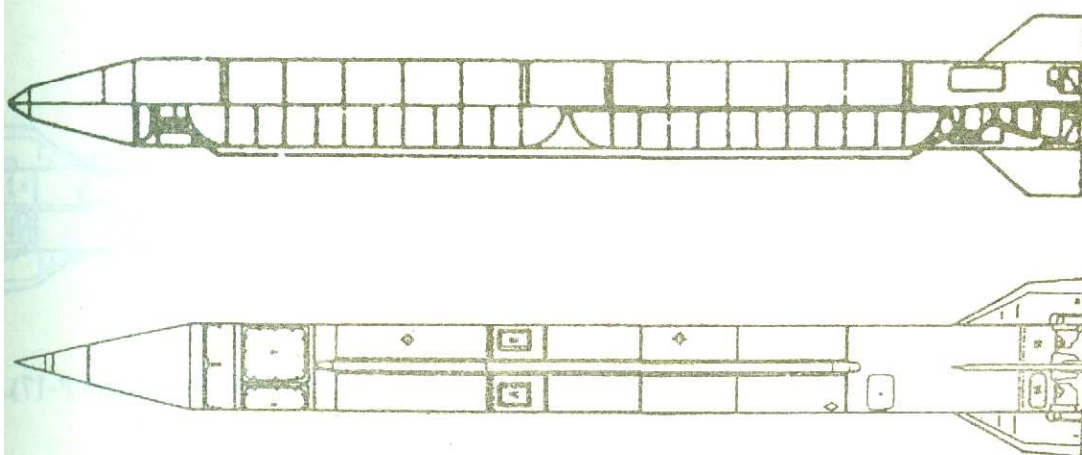
Ракета Р-17 комплекса 9K72 (SS-1c).
