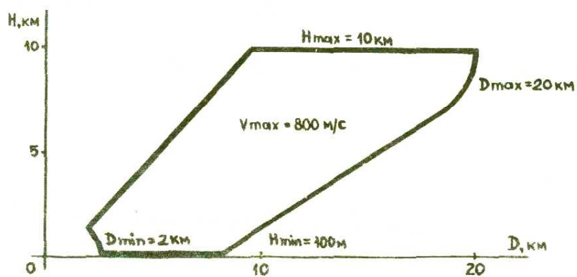
Зона возможных пусков ракет X-25MTП и X-25MT.
