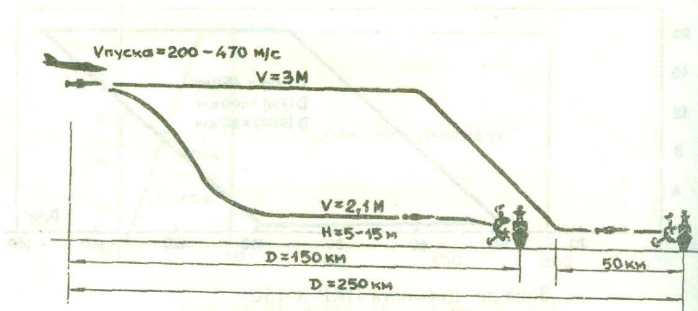
Схема боевого применения ракеты "Москит".
