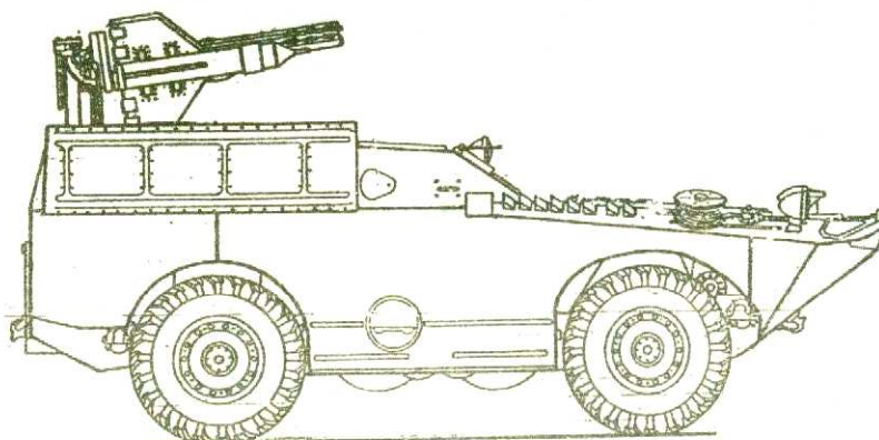
Боевая машина 2П27 с ПТУР 3М6(АТ-1).
