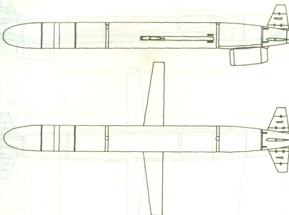
Авиационная ракета X-55 (AS-15A).
