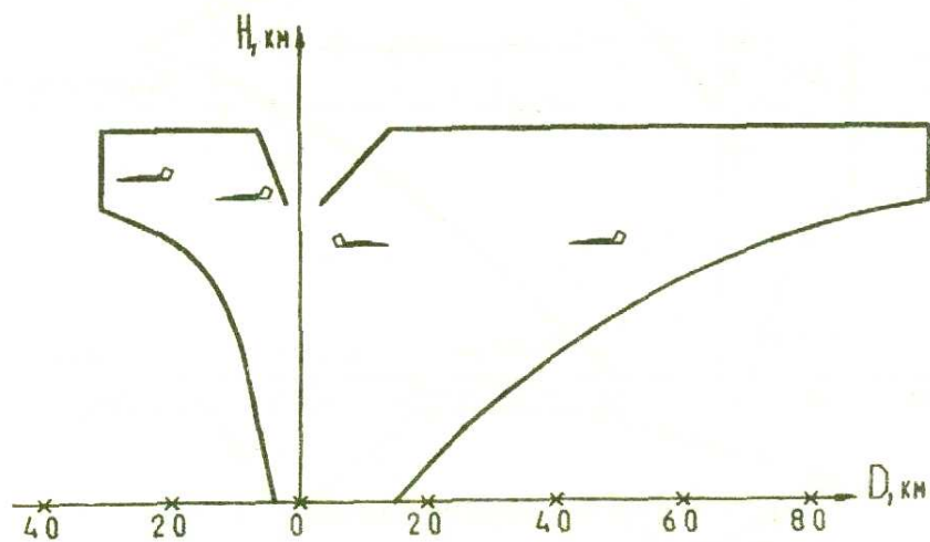
Схема боевого применения ракеты Р-77.
