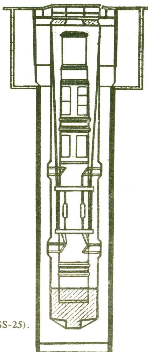
ШПУ ракетного комплекса РС-20, переоборудованная под ракетный комплекс "Тополь" (SS-25).
