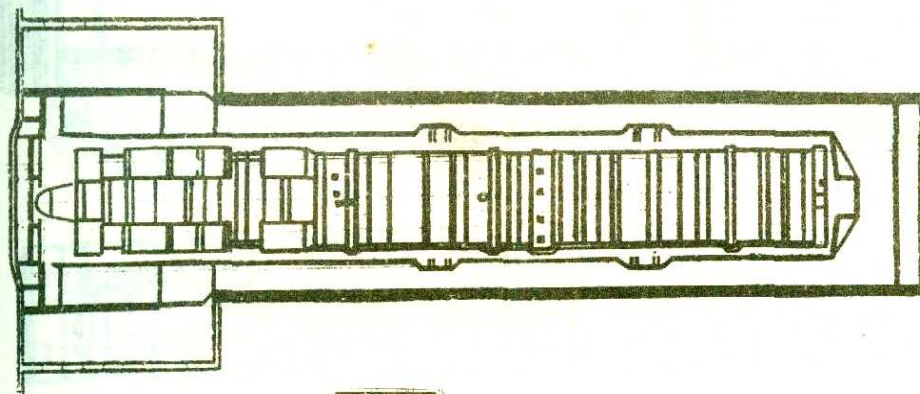
ШПУ ракетного комплекса РС-20 (SS-18).
