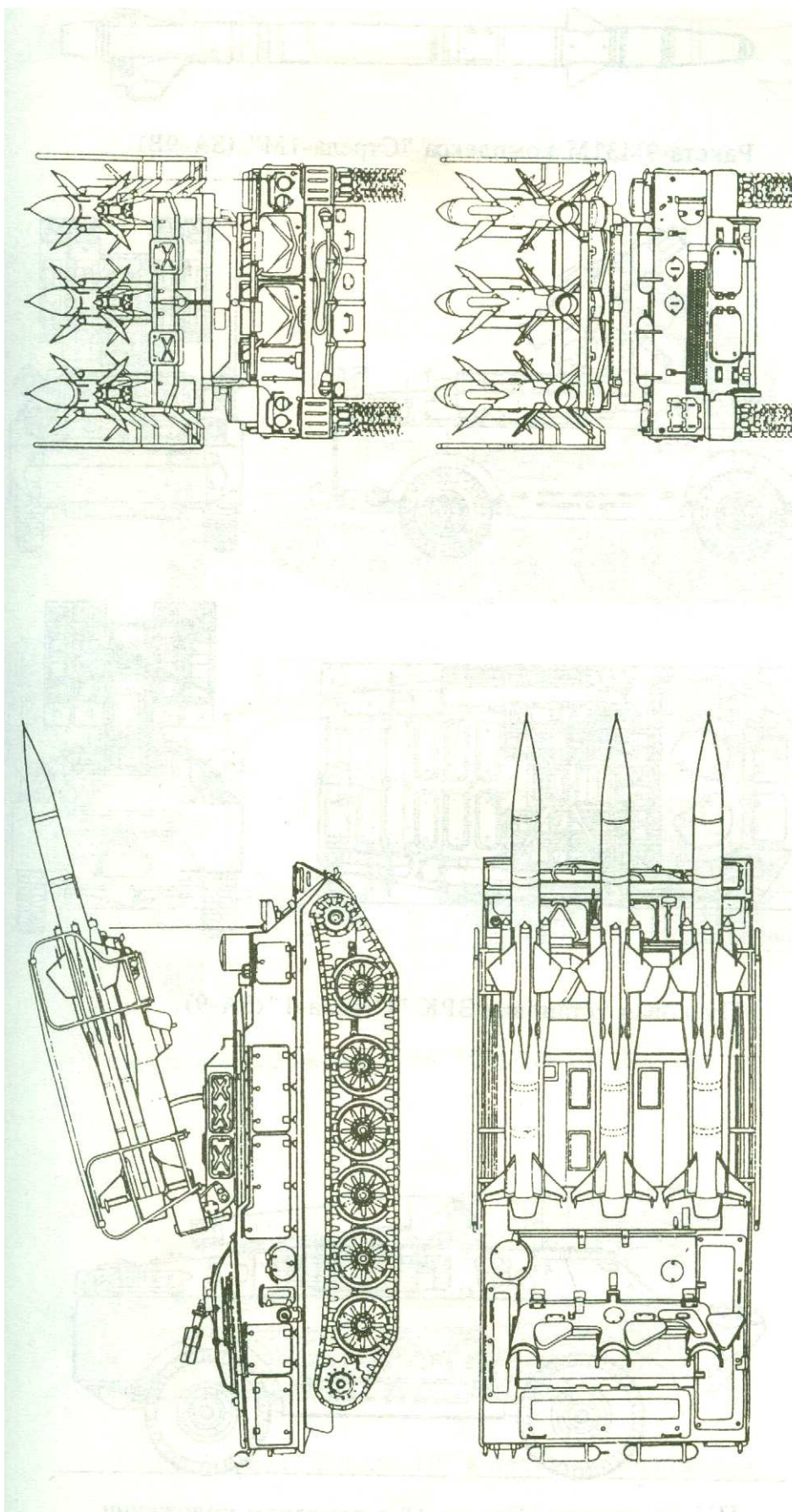
Пусковая установка с ракетами 3М8 комплекса "Куб" (SA-6).
