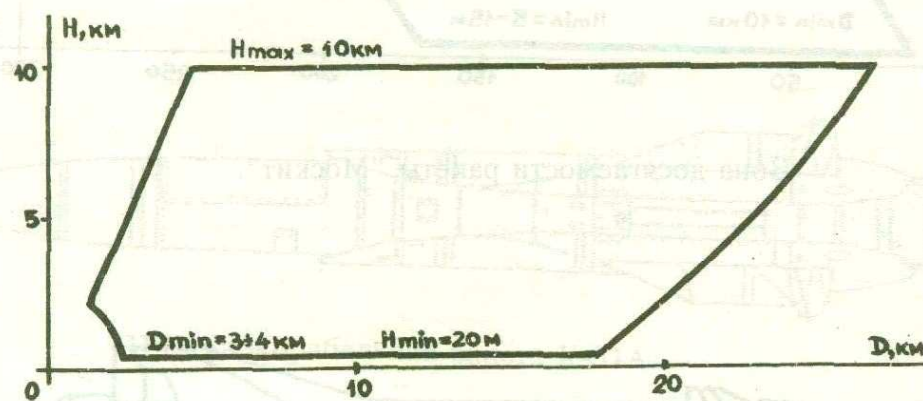
Зона возможных пусков ракеты Х-29Т (модернизированная).
