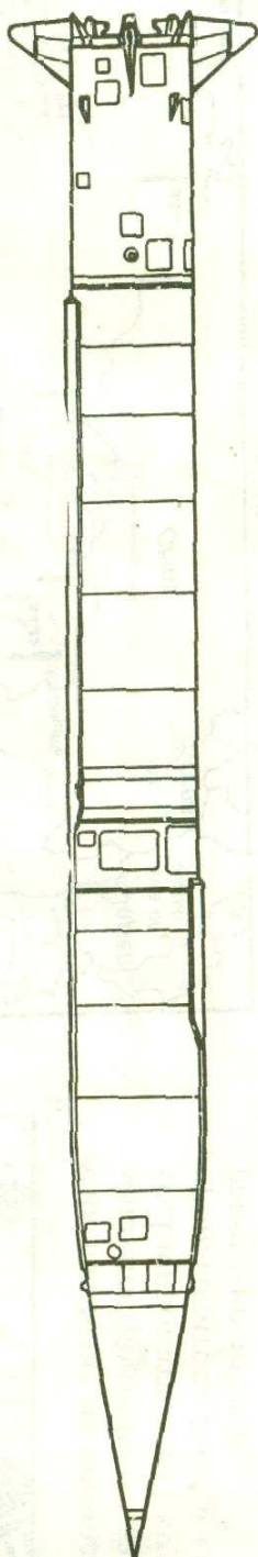
Баллистическая ракета Р-5 (SS-3).
