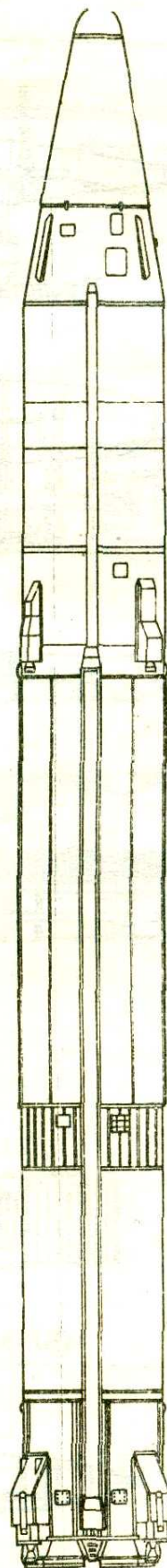
Внешний вид МБР Р-36 (SS-9).
