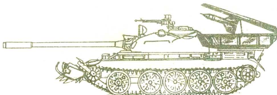
Танк Т-55 с ПТУРС 3М6 "Шмель" (АТ-1).
