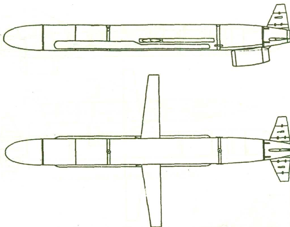
Авиационная стратегическая ракета РКВ-500Б (AS-15B).
