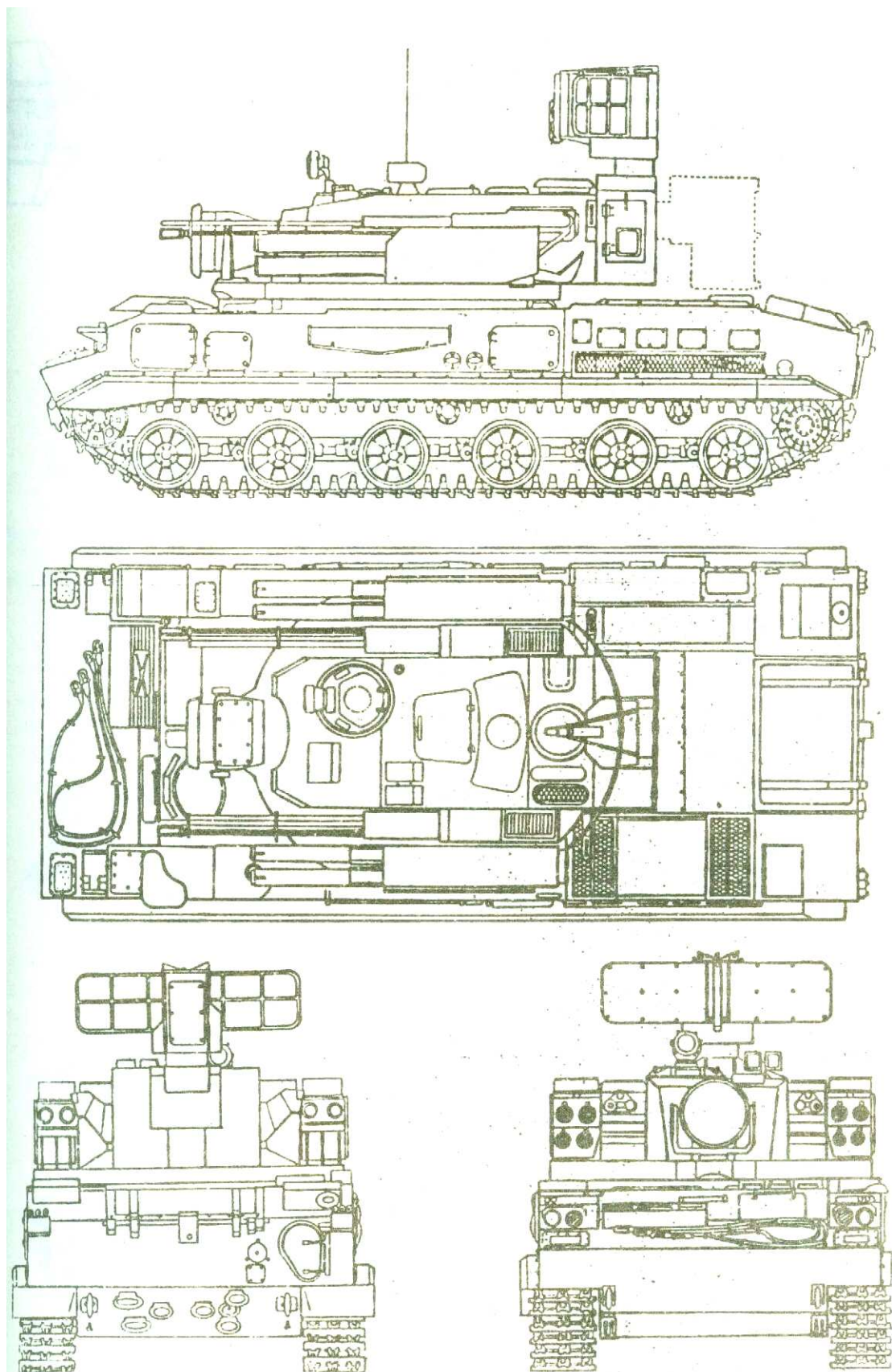
Боевая машина 2С6М комплекса 2К22М "Тунгуска" (SA-19).
