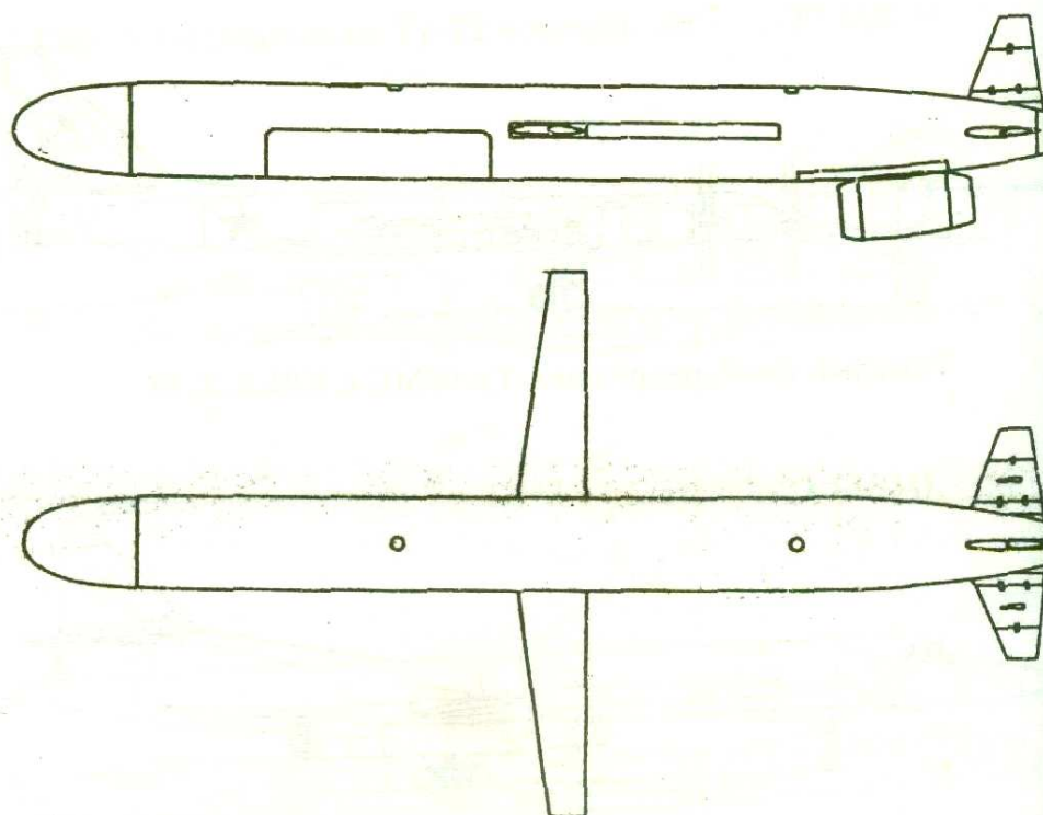
Оперативно-тактическая ракета типа X-55.
