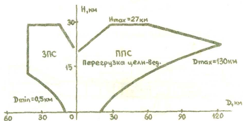
Зона возможных пусков ракеты Р-27АЭ.
