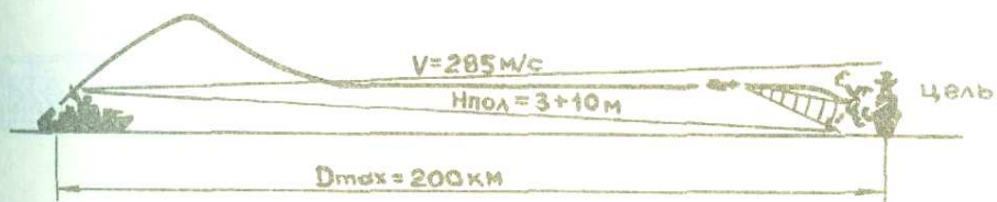
Схема боевого применения ПКР на базе X-59М.
