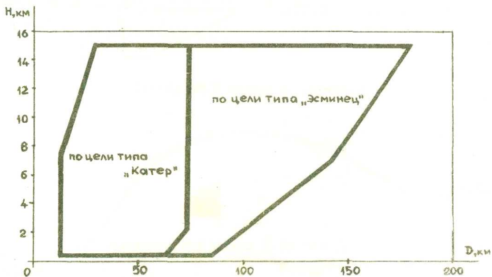
Зона досягаемости ПКР на базе Х-58.
