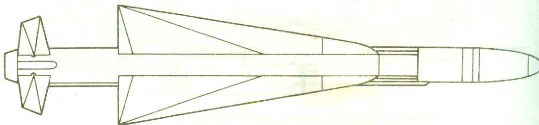
Истребитель-перехватчик Ту-128 с ракетами Р-4Р и Р-4Т.
