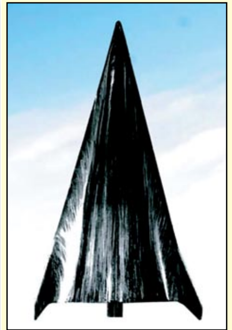
Маслосажежая картина линий тока на поверхности модели ELAC 1, полученная в аэродинамической трубе T-313 Института теоретической и прикладной механики СО РАН.
