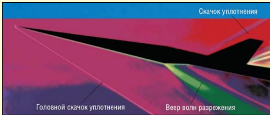
Эта теневая картина обтекания модели ELAC 1 получена оптическим методом Теплера в сверхзвуковой аэродинамической трубе в Ахене
