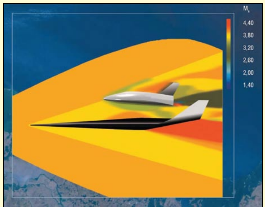
Теоретическое распределение чисел Маха (скоростей) при обтекании двухступенчатой конфигурации ELAC–EOS (число Маха набегающего потока M = 4,04 )
