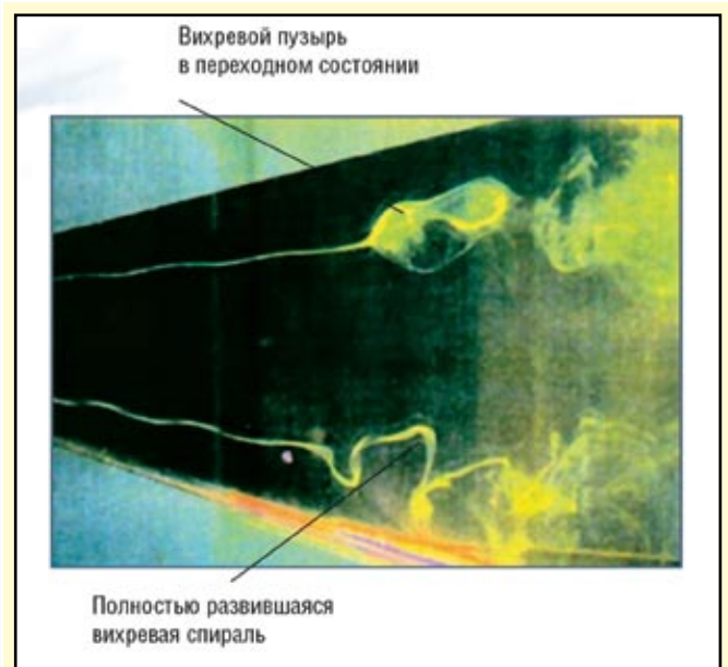
Процессы распада вихрей на подветренной стороне конфигурации ELAC 1 визуализировались посредством впрыска флуоресцентной краски
