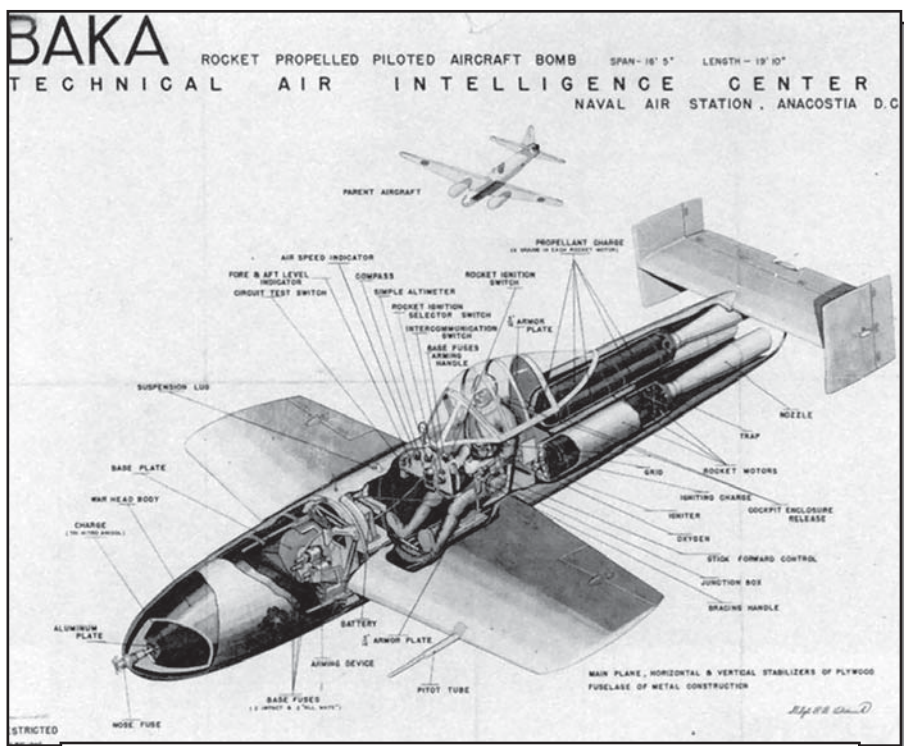
Для ознакомления с конструкцией ракетного самолета для камикадзе разведслужба ВМС США подготовила такой плакат. Фото: архив автора
