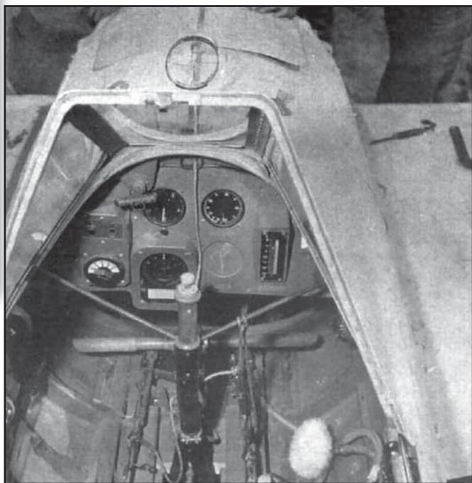
В кабине самолета-снаряда МХУ7 «Ока» Модель 11 было установлено лишь самое необходимое оборудование
