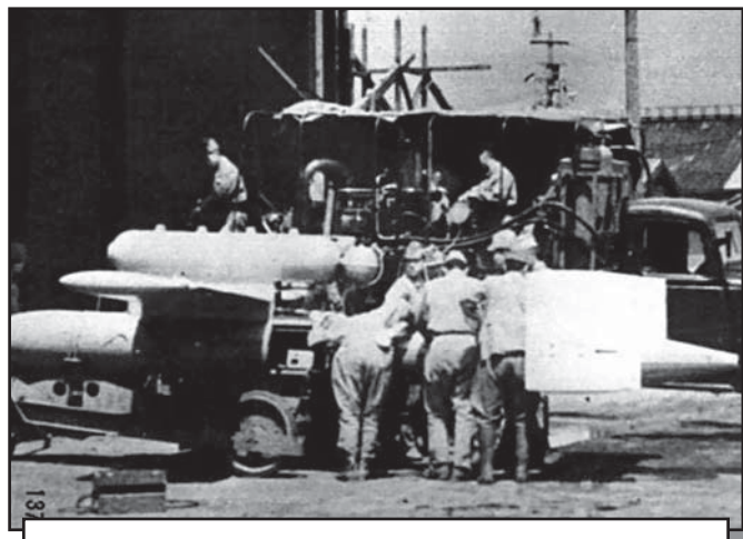
Управляемая ракета Мицубиси Ки 147 «И-Го» Тип 1-а (1-Ко) на транспортировочной тележке готовится к подвеске на самолет Ки 67-1 GO-IA «Хириу», 1945 г.
