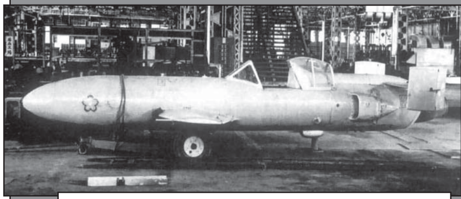
Самолет-снаряд МХУ7 «Ока» Модель 22 с мотокомпрессорным воздушно-реактивным двигателем был рассчитан на повышенную дальность
