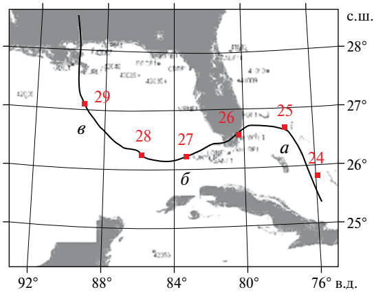
Карта движения тропического урагана Катрина 24–29 августа 2005 г. (слева). Графики вариаций яркостной температуры в системе океан–атмосфера ( \lambda = 1,26 см), измеренные с помощью радиометра AMSR-E ИСЗ “Аква” в различных точках траектории продвижения урагана от очага его возникновения – к южному побережью США: а) 26° с.ш., 78° з.д.; б) 25° с.ш., 83° з.д.; в) 27° с.ш., 89° з.д. (справа). Наблюдается перемещение всплесков яркостной температуры, совпадающее с траекторией распространения урагана.
