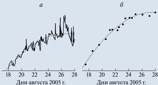
Графики нарастания приводной влажности воздуха (по данным станции SMKF1 (а) и яркостной температуры системы океан–атмосфера на длине волны 1,26 см (на основании данных, полученных с помощью радиометра AMSR-E ИСЗ “Aqua” (б) в августе 2005 г. Кривыми показан постепенный рост показателей.
