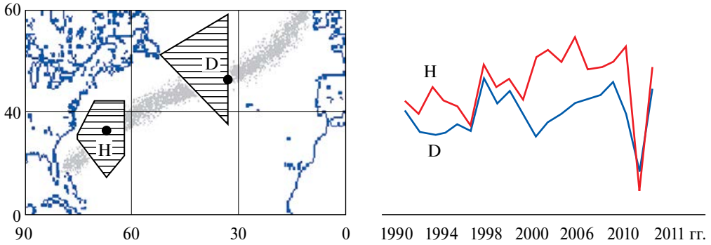
Карта течения Гольфстрим и энергоактивные области (H) и (D) на его пути (слева). График динамики изменений общего содержания водяного пара в атмосфере и его особенности в 2010 г. (справа). Отмечается значительное снижение среднегодовых значений общего содержания водяного пара в атмосфере в Ньюфаундлендской (D) и Гольфстримской (H) областях после начала нефтяных разливов в мае 2010 г.
