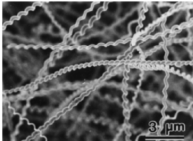
8 Электронная микрофотография спиралевидных нановолокон, образующих «углеродную резину»
