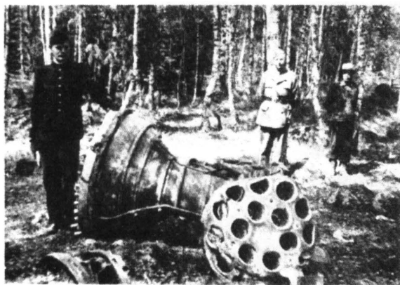
Fig. 8. Reaktionsaggr., huvudbrännaren
