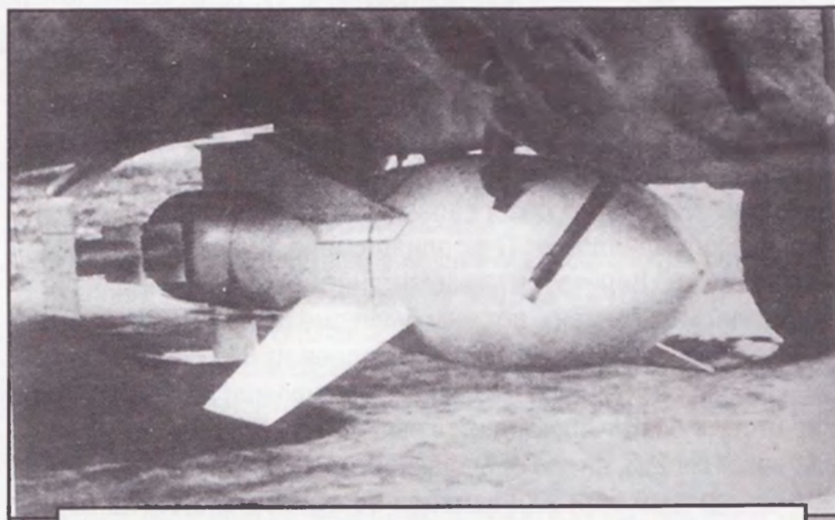
Подвеска управляемой планирующей бомбы «Фриц-X» под самолет-носитель He 177A-5 «Грайф»
