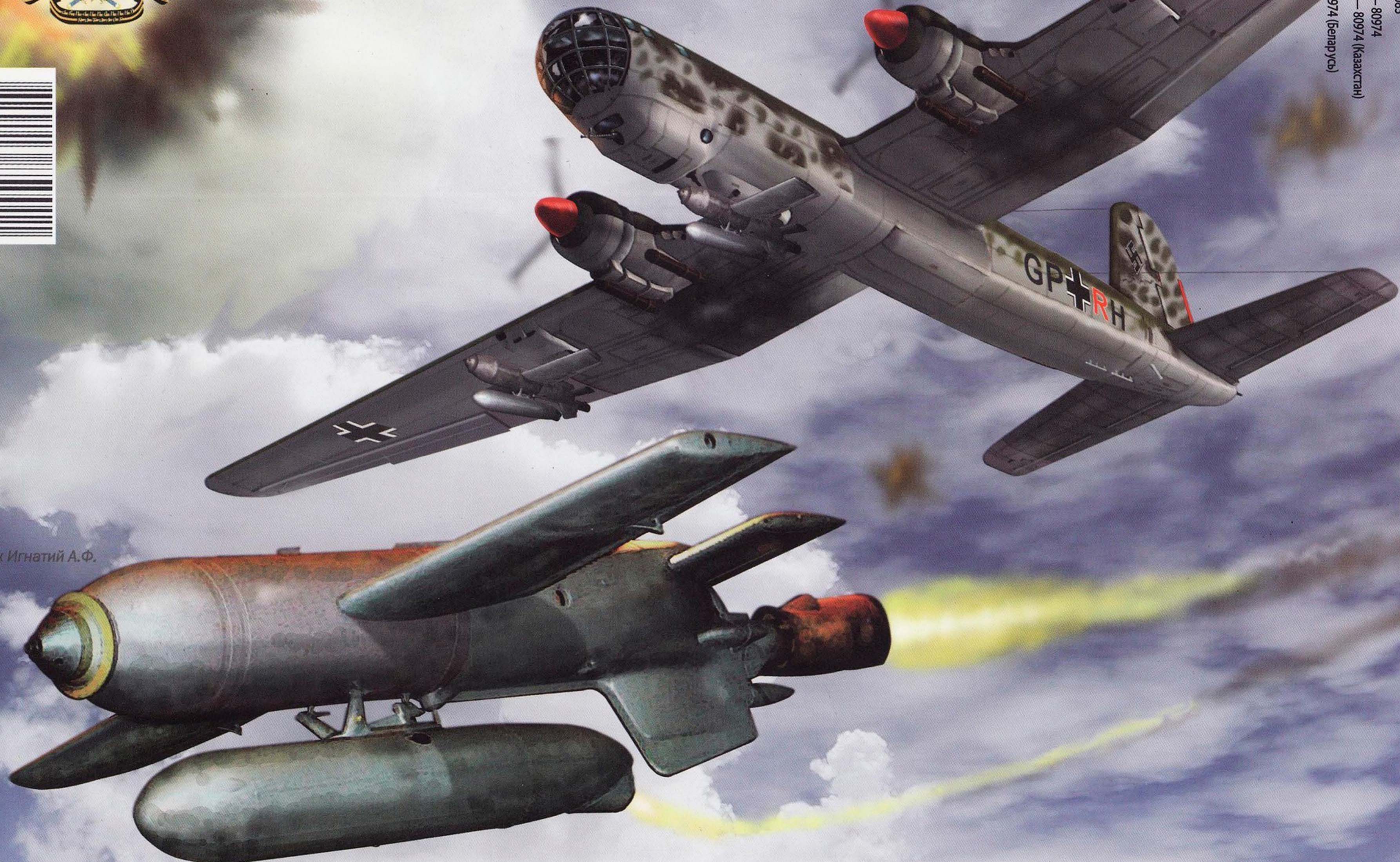
Пуск противокорабельной ракеты Hs 293A-1 бомбардировщиком He-177A
