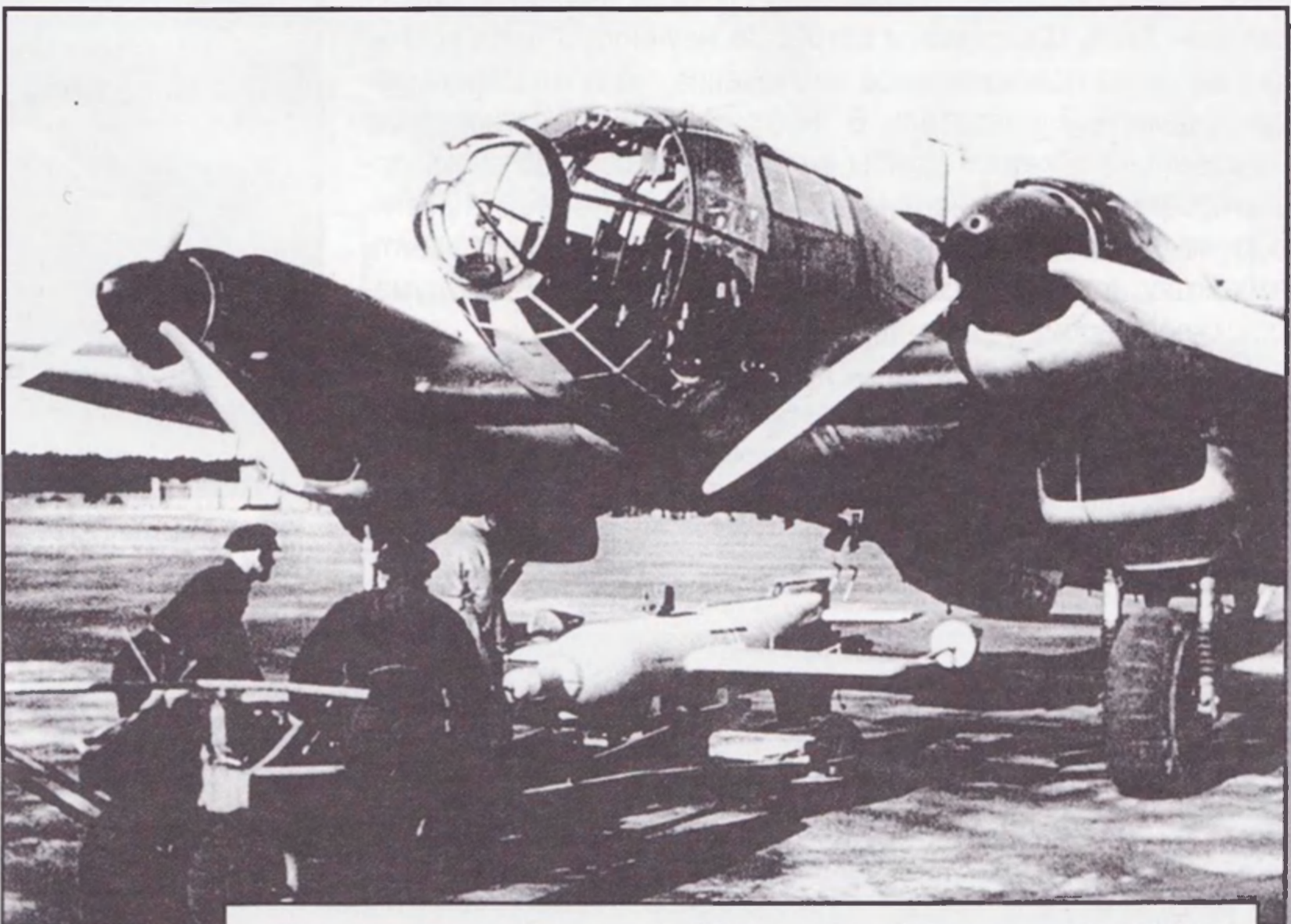
Подвеска ракеты Хеншель Hs 293A-0 на бомбардировщик He 111Н
