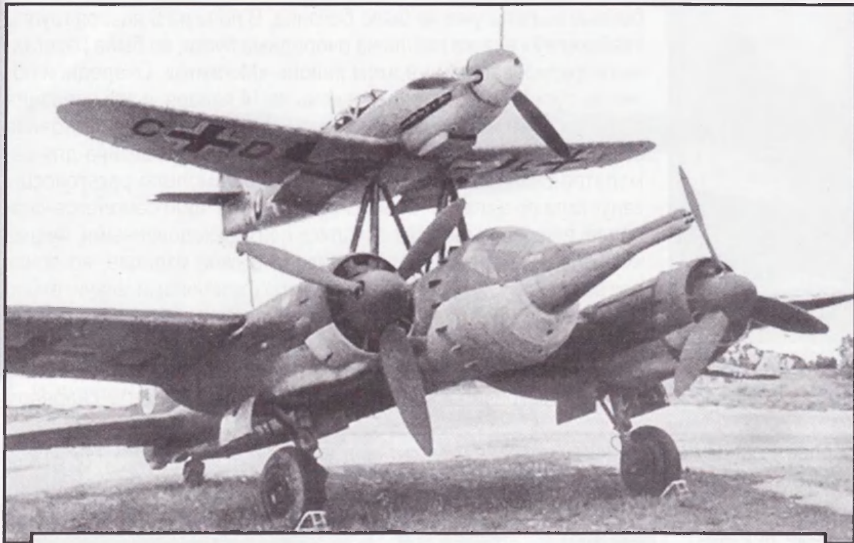
«Мистель 1», самолет-бомба Юнкерс Ju 88А-4 и самолет управления Мессершмитт Bf 109F, задумывалась как стратегическая наступательная, но использовалась лишь для разрушения мостов перед наступающими войсками Союзников
