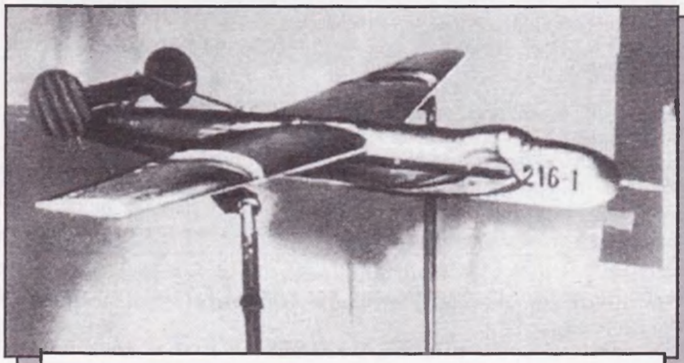
Крылатая ракета воздушного старта «216» конструкции С.П. Королева в аэродинамической трубе
