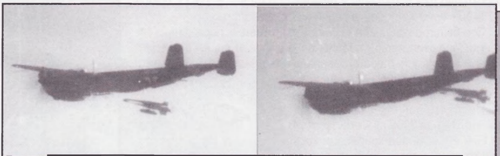
Кинокадры испытательного пуска усовершенствованной ракеты Hs 294 с отделяемой боевой частью с борта Do 217
