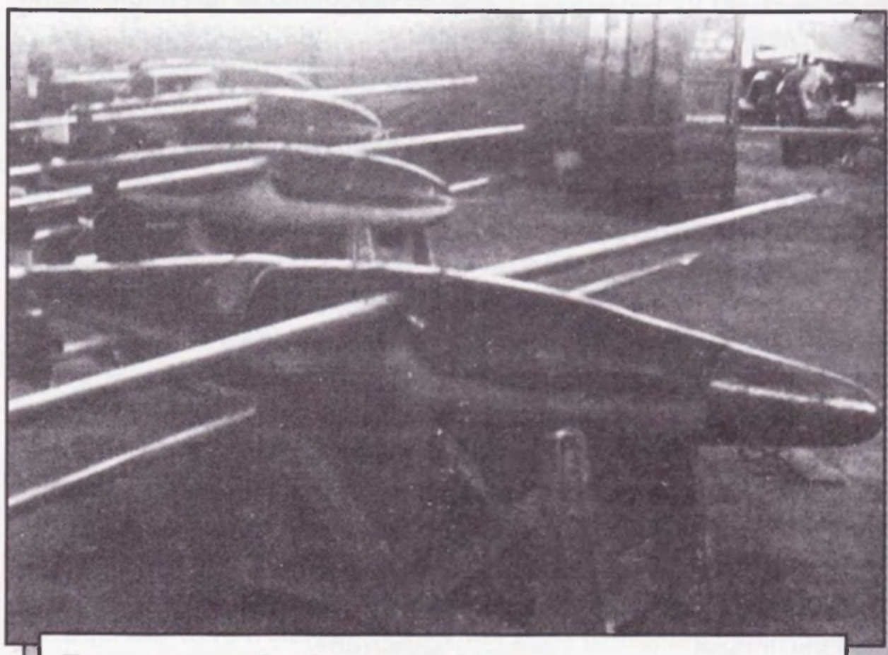
Планирующая бомба BV 246 «Радизшен» — вариант с пассивной противорадиолокац. системой самонаведения
